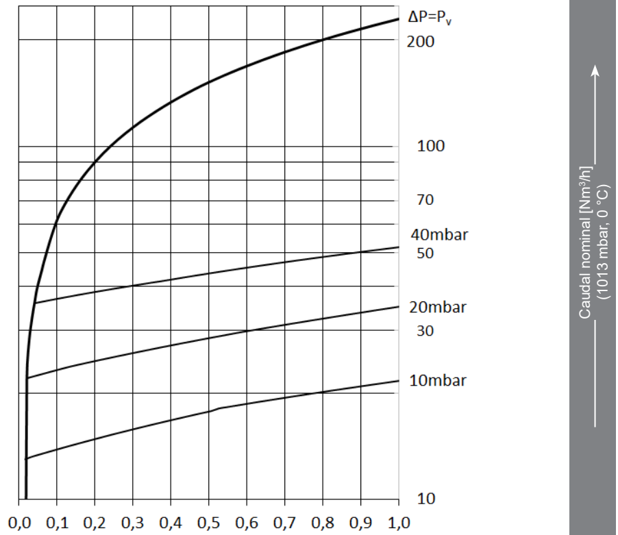
Diagrama de caudal para aire (20 °C)
