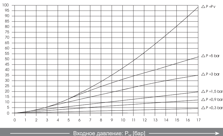
Диаграмма пропускной способности для водорода (20 °C)
