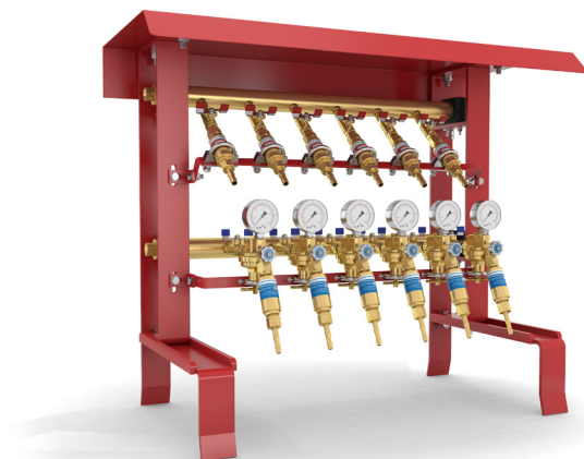
mit 4 oder 6 Entnahmestellen und bis zu 5 verschiedenen Gasarten Universal 704
