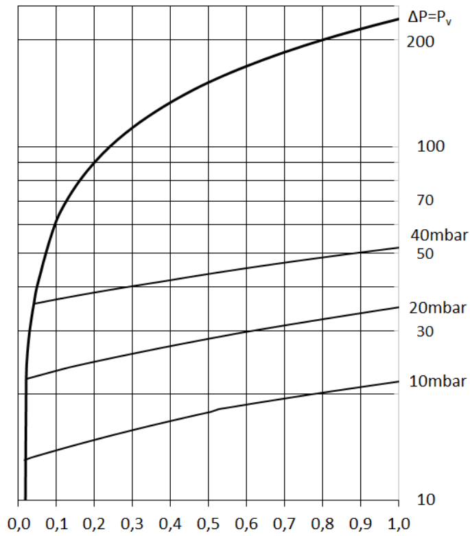
Durchflussdiagramm für Luft (20 °C)
