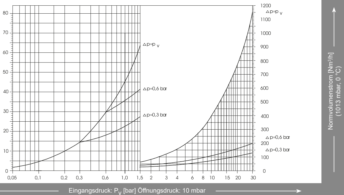
Durchflussdiagramm für Luft (20 °C)
